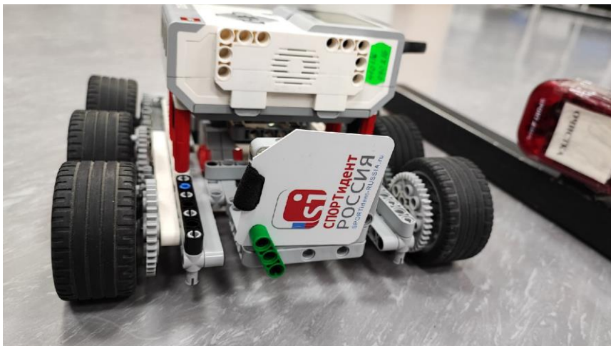
Рисунок 3. Вариант установки ЧИПа на роботе.
